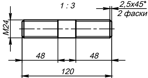
Поз.6 (Шпилька) 1 : 3
