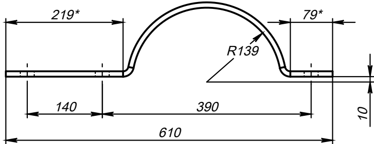
Поз.5 (Полухомут) развертка
