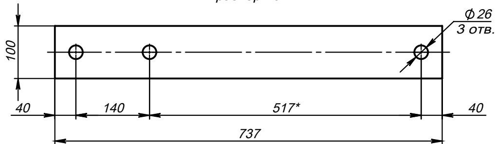
Поз.5 (Полухомут) развертка
